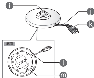
電源ベース
